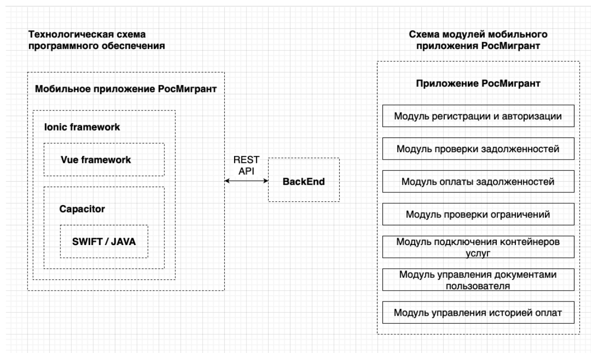
Рис. 1. Общая схема ПО
